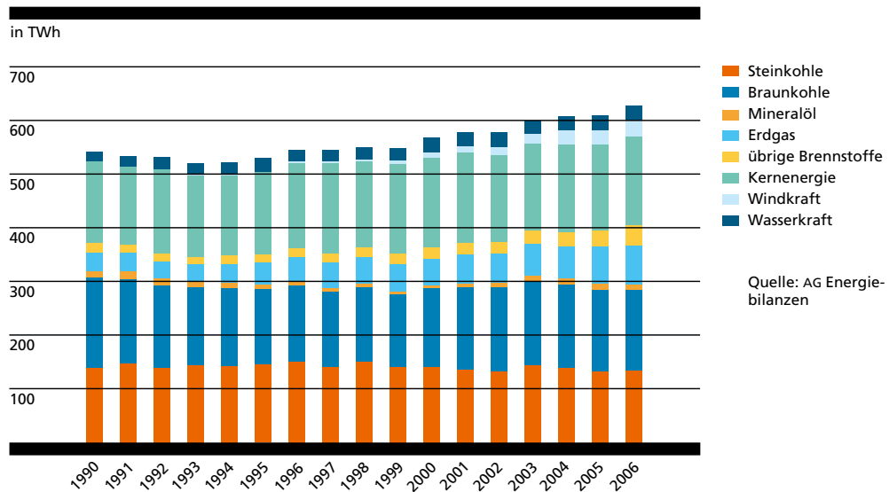
BRUTTOSTROMERZEUGUNG NACH ENERGIETRÄGERN IN DEUTSCHLAND (ABB. 5)
