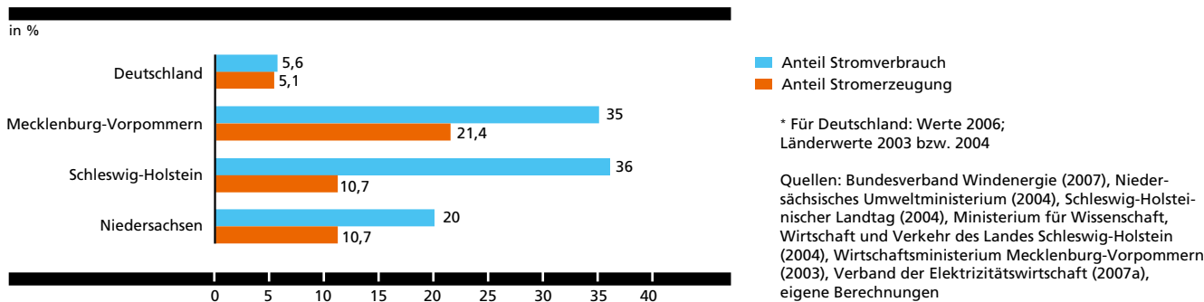
ANTEIL DES MIT WINDENERGIE ERZEUGTEN STROMS AM STROMVERBRAUCH UND AN DER STROMERZEUGUNG 2003–2006* (ABB. 12)
