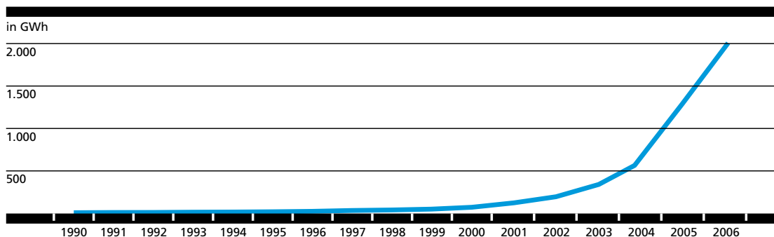
STROMERZEUGUNG MIT PHOTOVOLTAIK IN DEUTSCHLAND 1990–2006 (ABB. 14)
