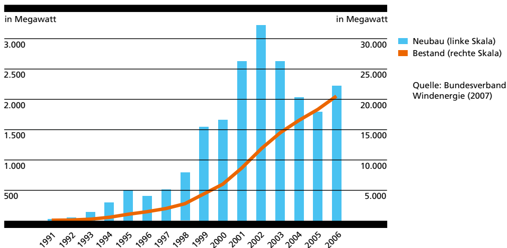
WINDENERGIE IN DEUTSCHLAND – NEUBAU UND BESTAND (ABB. 13)
