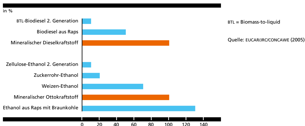
CO 2 -AUSSTOSS VON BOKRAFTSTOFFEN IM VERHÄLTNIS ZUM MINERALISCHEN KRAFTSTOFF (ABB. 11)
