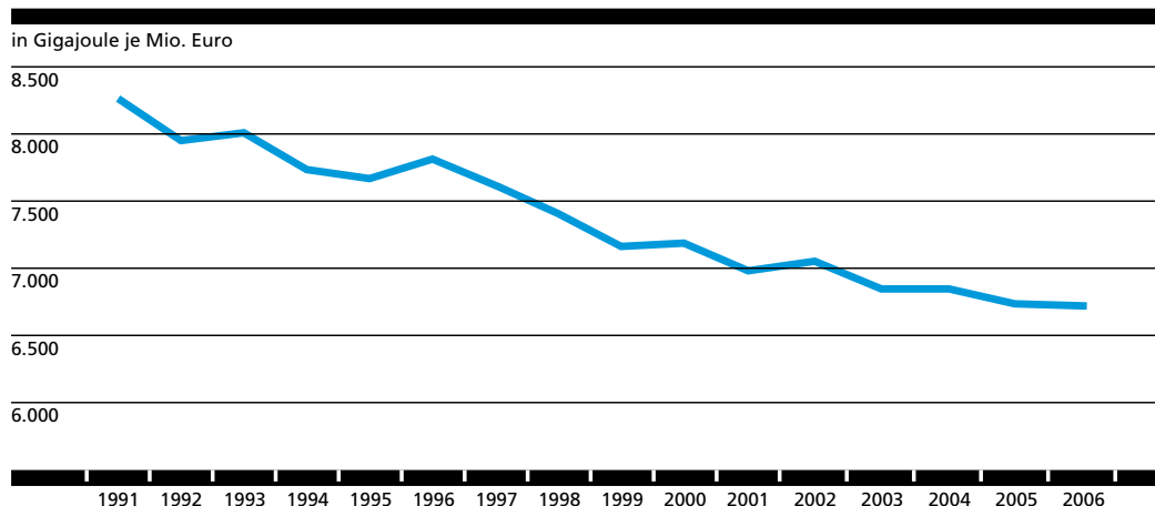
ENTWICKLUNG DER ENERGIEINTENSITÄT IN DEUTSCHLAND 1991–2006 (ABB. 19)
