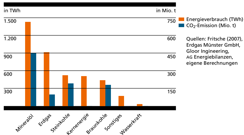
PRIMÄRENERGIEVERBRAUCH UND CO 2 -EMISSIONEN NACH ENERGIETRÄGERN 2006 (ABB. 3)
