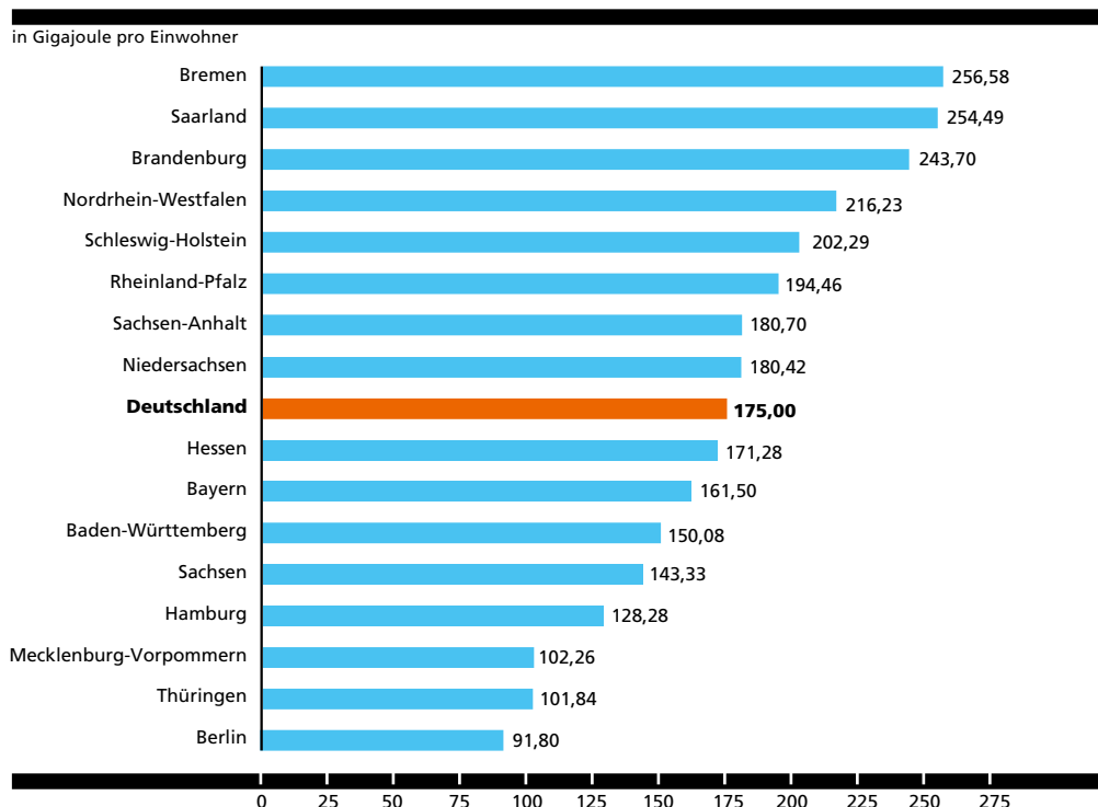
PRIMÄRENERGIEVERBRAUCH PRO EINWOHNER NACH BUNDESLÄNDERN 2004* (ABB. 4)
