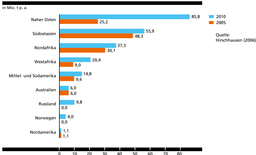
WELTWEITE VERFLÜSSIGUNGSKAPAZITÄTEN VON ERDGAS (ABB. 22)
